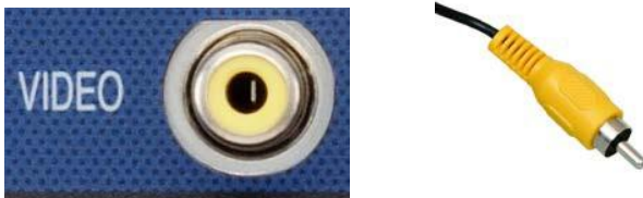
Connectique RCA
